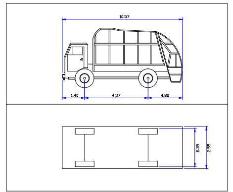
Standardi France, Name: Camion déchets ménagers, Total length: 10.57(m)
